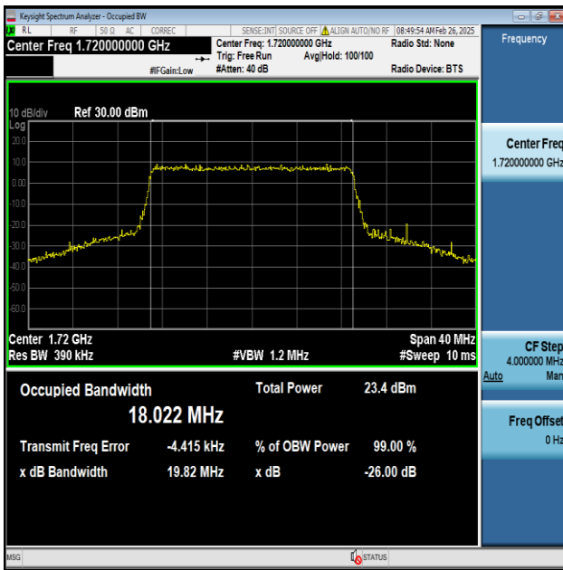
Band4-20MHz-QPSK-20050-100RB#0-PASS
