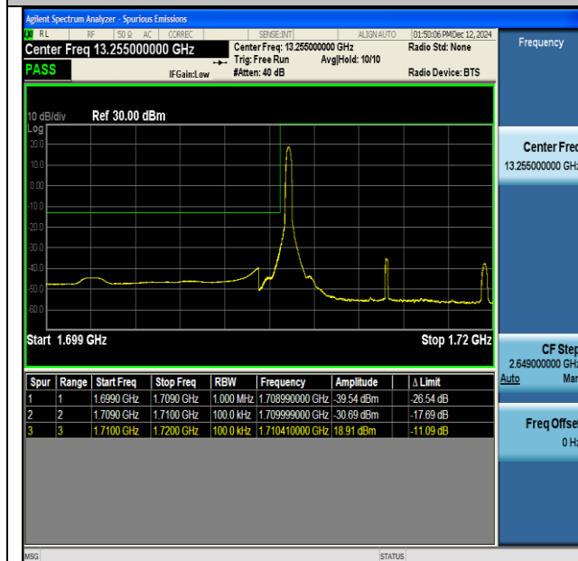
NTNV-DC_13A_n66A-PC3-15-5+10-M+L-QPSK-IDLE-CP- QPSK-Edge_1RB_Left-PASS
