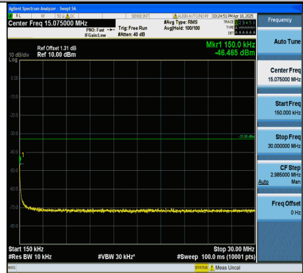
GPRS1900-661-0-0.15~30MHz-PASS
