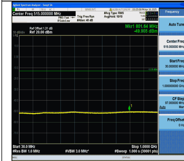
GPRS1900-661-0-30~1000MHz-PASS
