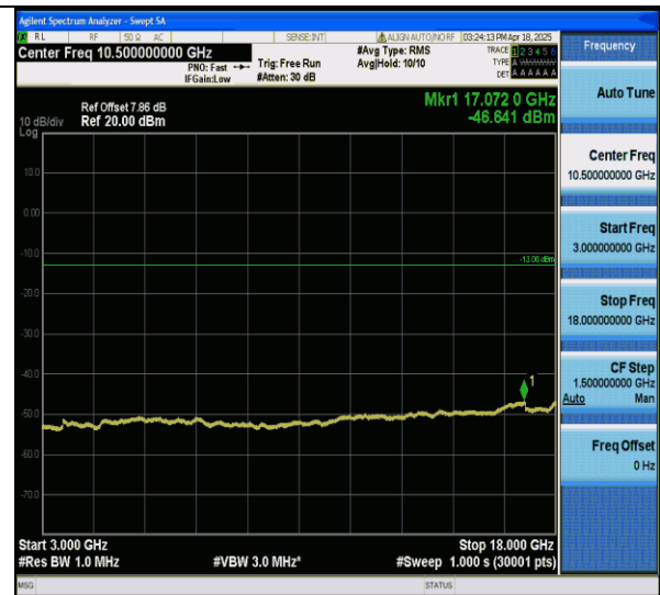
GPRS1900-512-0-3000~18000MHz-PASS
