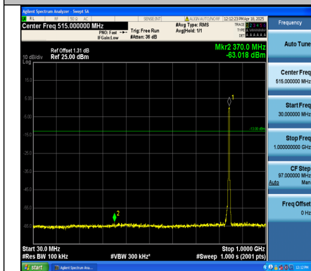
Band V-4233-30~1000MHz-PASS
