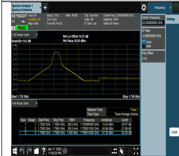
Band4-20MHz-QPSK-20300-1RB#99-PASS
