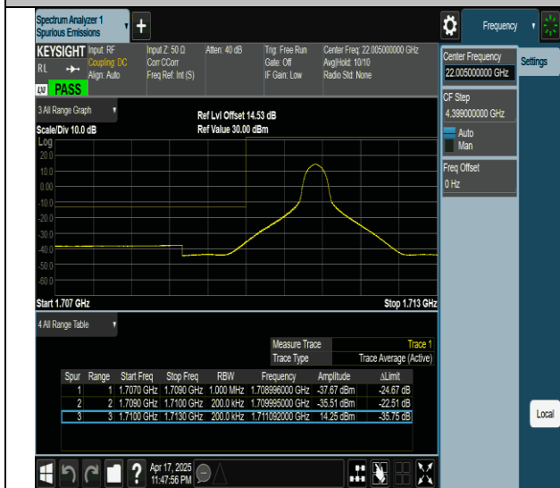
Band4-20MHz-QPSK-20050-1RB#0-PASS
