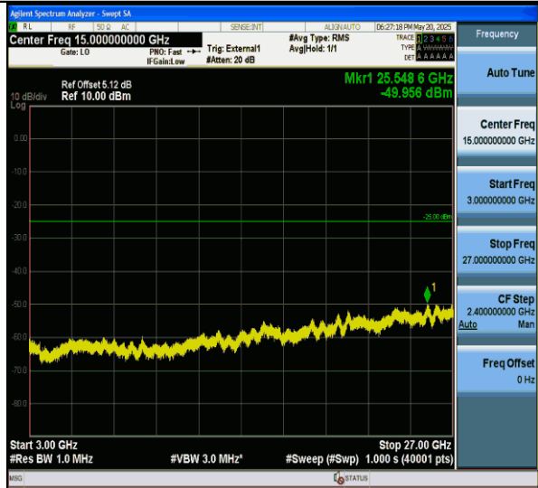
Band41-20MHz-QPSK-41490-1RB#0-3000~27000-PASS
