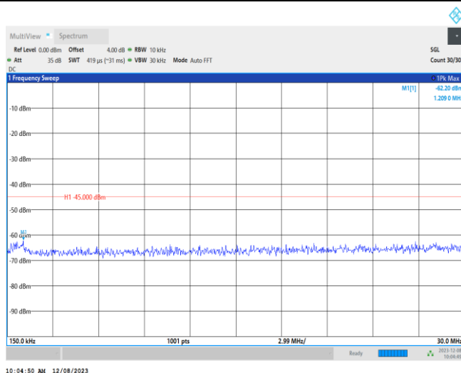
Band41-20MHz-QPSK-39750-1RB#0-Range2:0.15~30MHz
