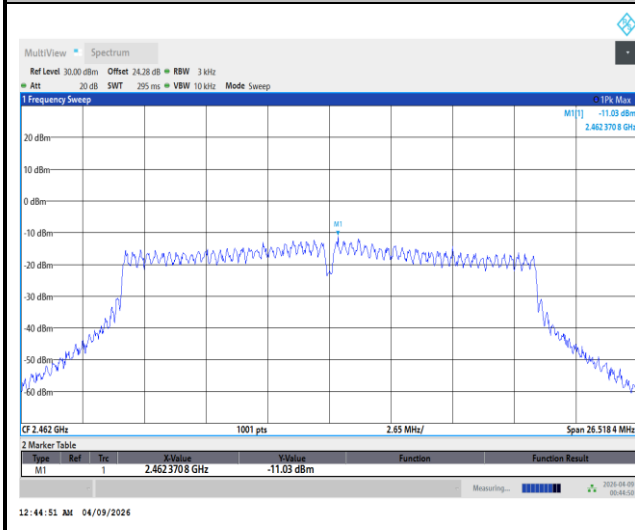
MIMO Ant. 6
