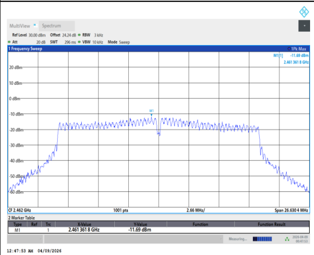
MIMO Ant. 7
