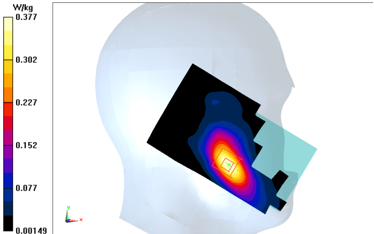
Fig.19 LTE Band7
