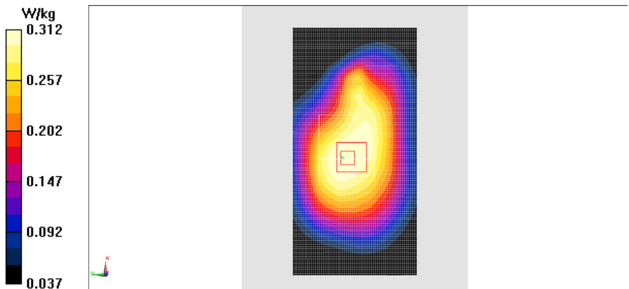
Fig.18 LTE Band5
