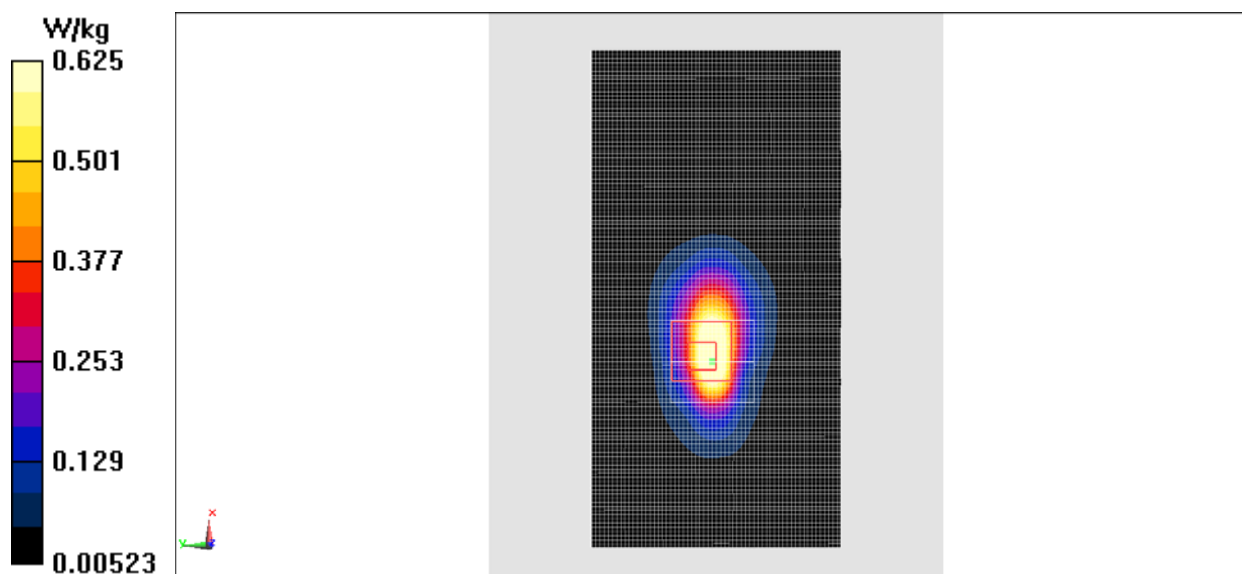
Fig.11 WCDMA1900
