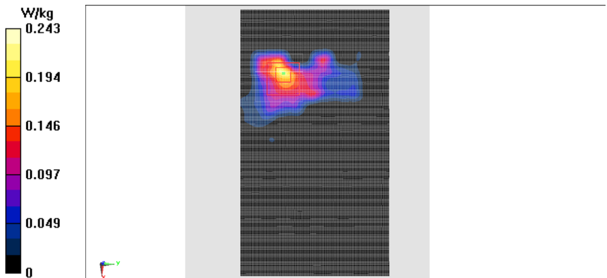
Fig.31 5GHz
