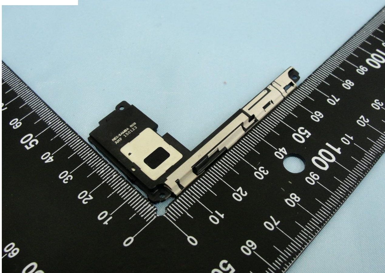
WWAN Antenna
