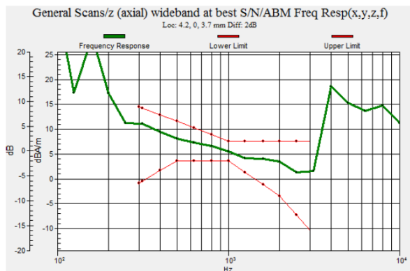
Fig 7.1 GSM850 Ch189
