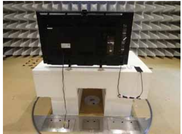
MHL mode
