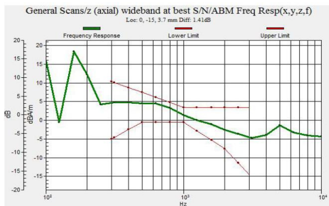
Fig 7.3 WCDMA Band II Ch9400
