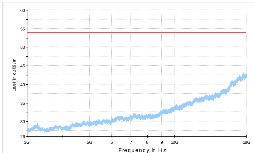
RE - 3GHz-18GHz
