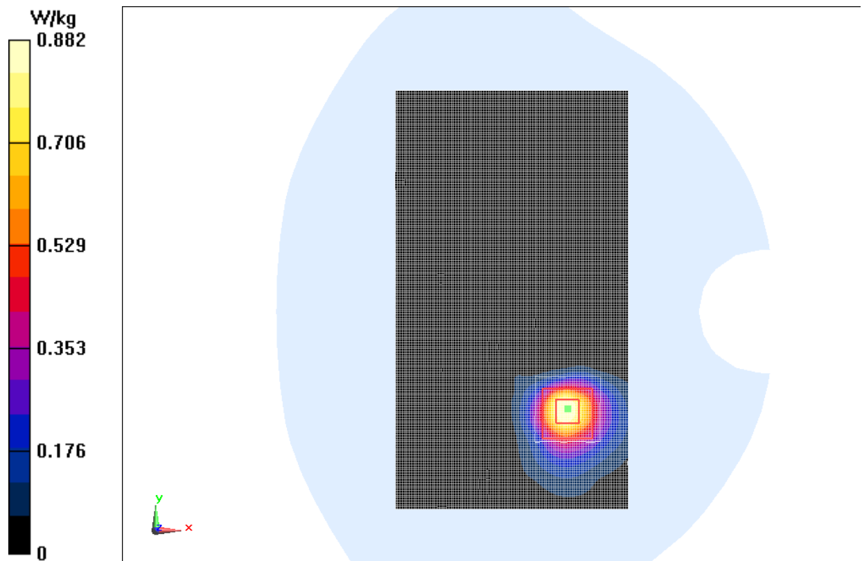
Fig.32 5GHz CH42
