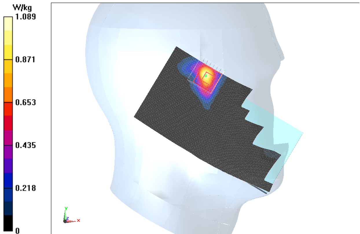
Fig.31 5GHz CH42
