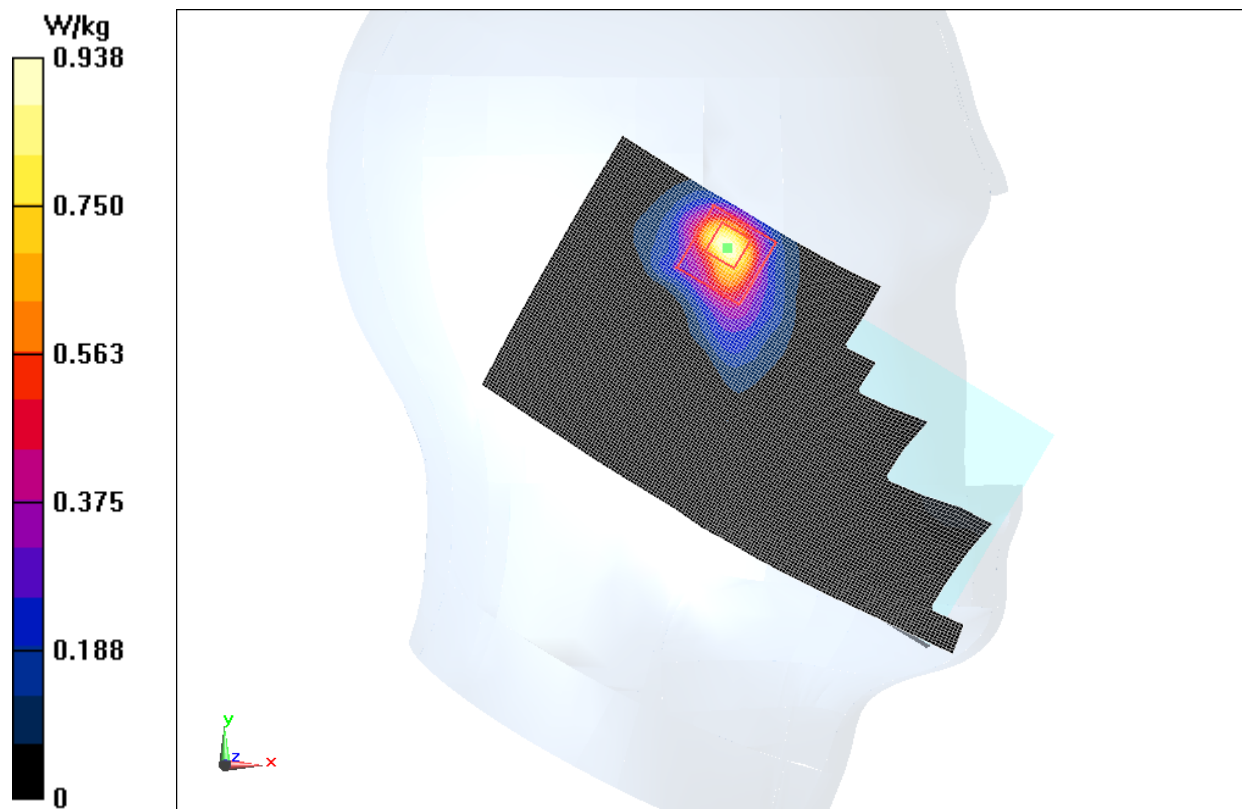
Fig.25 5GHz CH60
