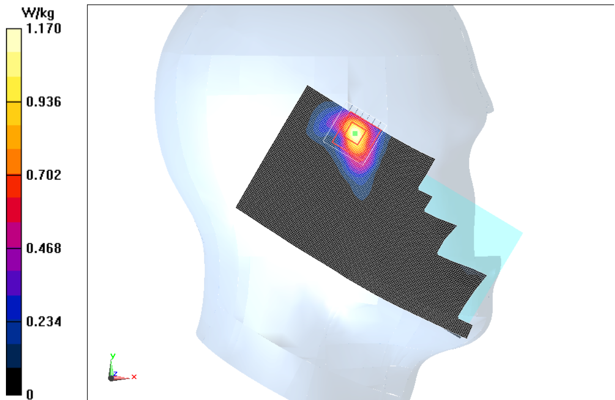
Fig.27 5GHz CH60
