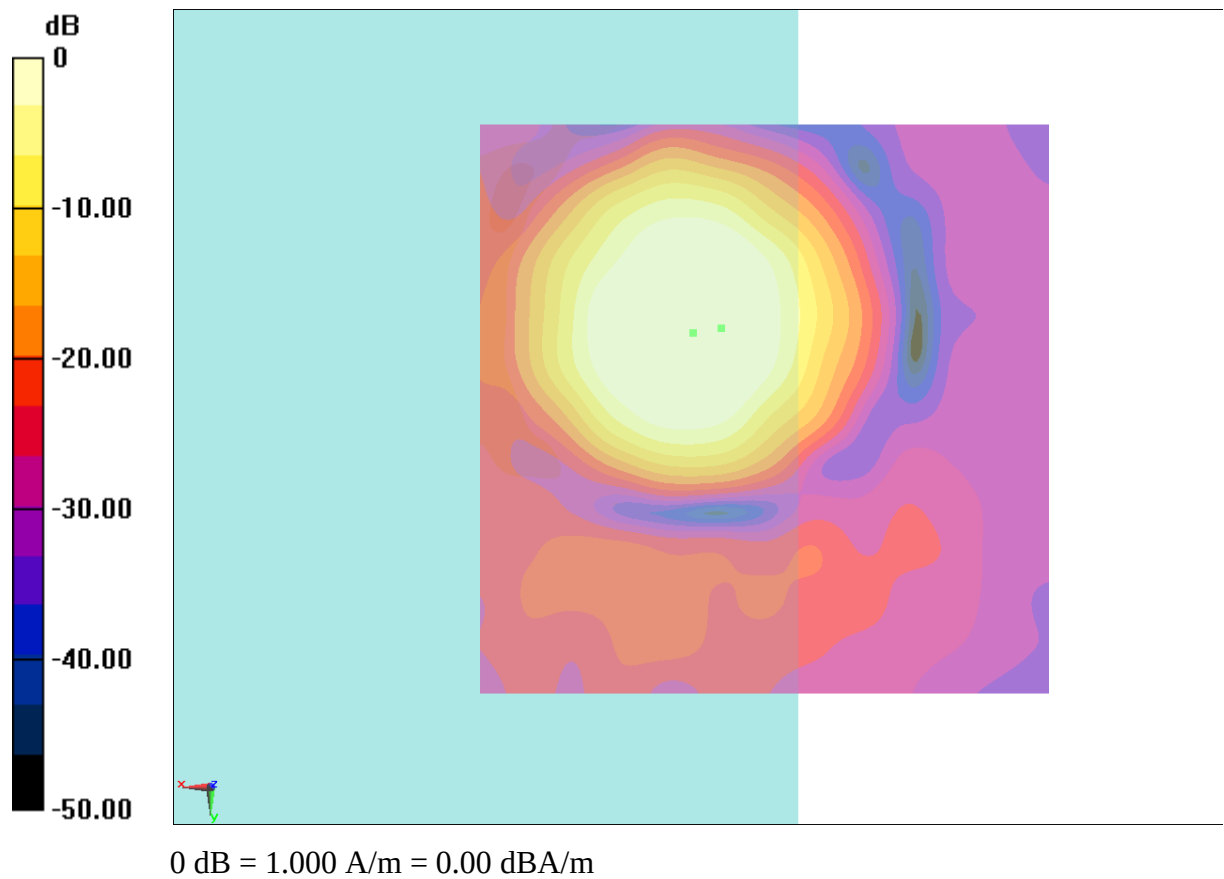
Fig B.4 T-Coil CDMA 835_Channel 384
