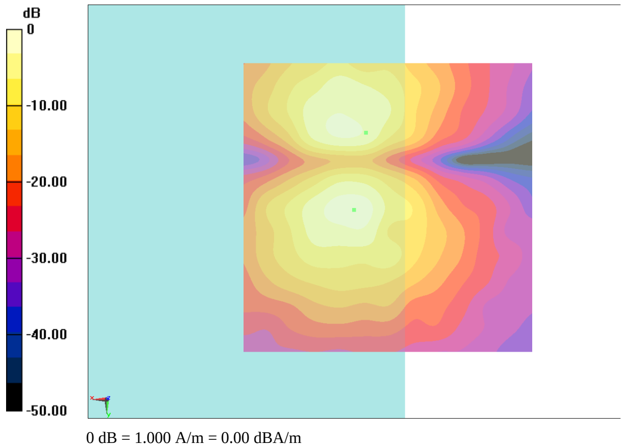
Fig B.3 T-Coil CDMA 835_Channel 384
