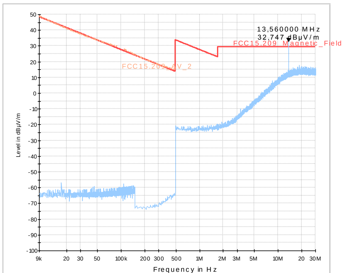
FCC15.209_magn hor+vert
