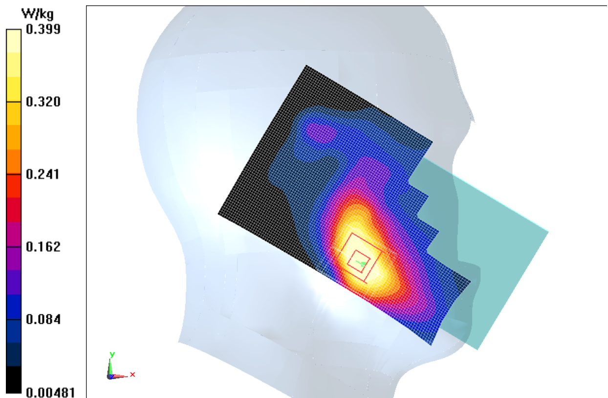
Fig.7 1700MHz CH1312
