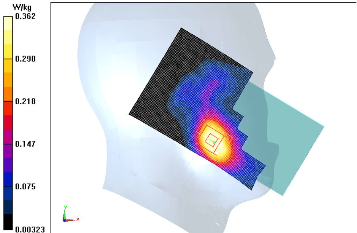
Fig.10 WCDMA1900 CH9400
