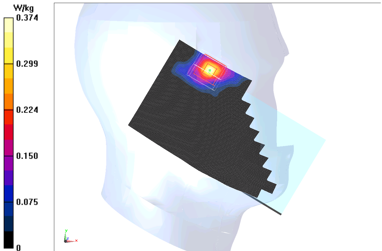
Fig.24 5GHz CH48
