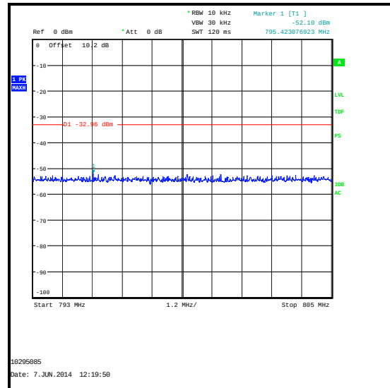
QPSK / 1 Resource Block 2450 Offset)
