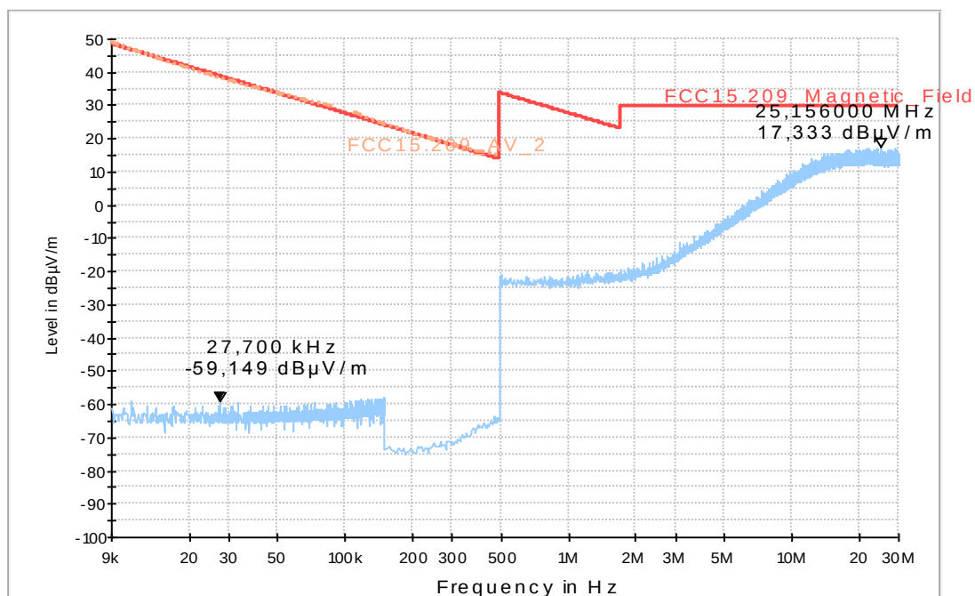
FCC15.209_magn hor+vert
