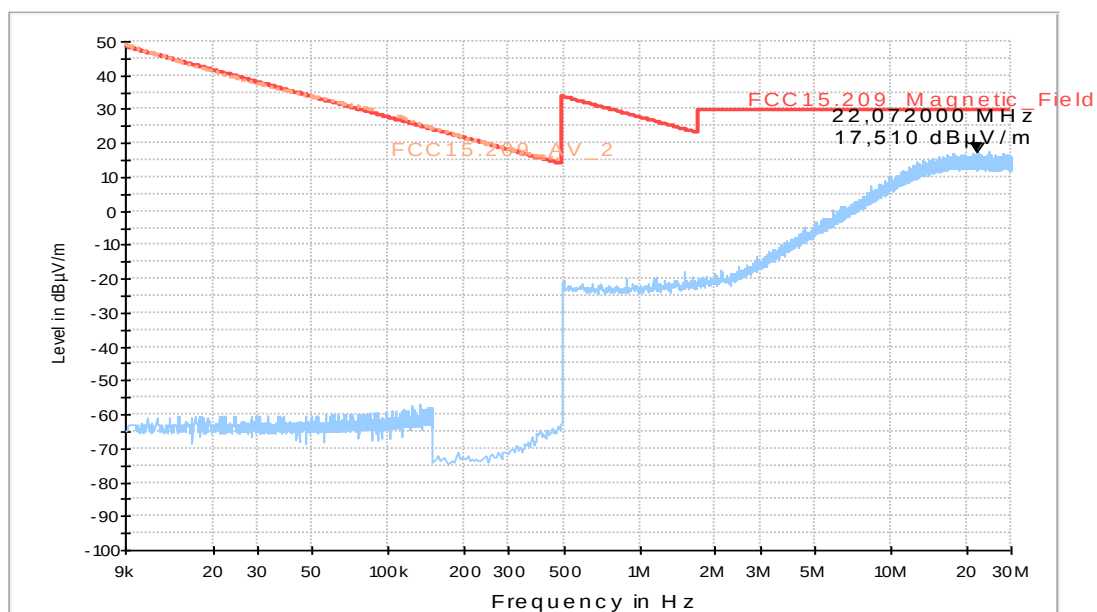
FCC15.209_magn hor+vert
