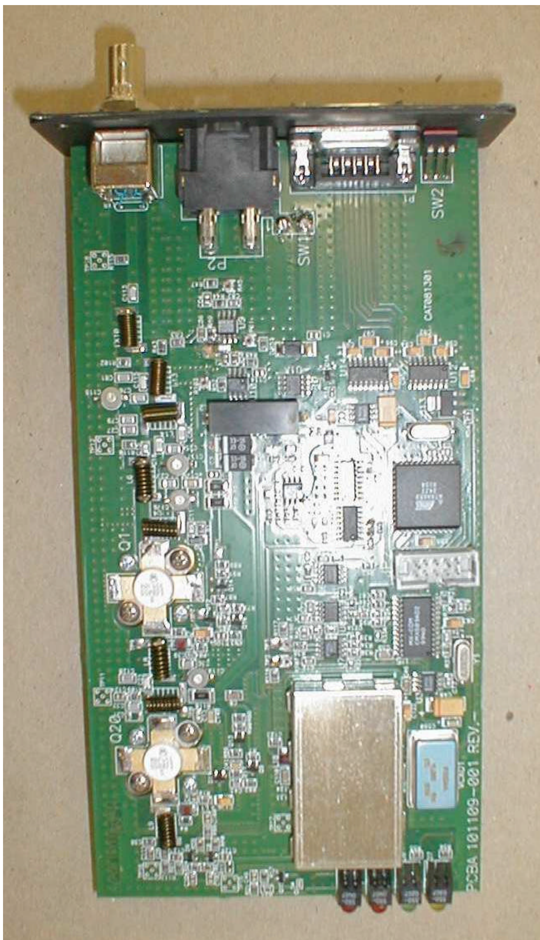
PCB Top
