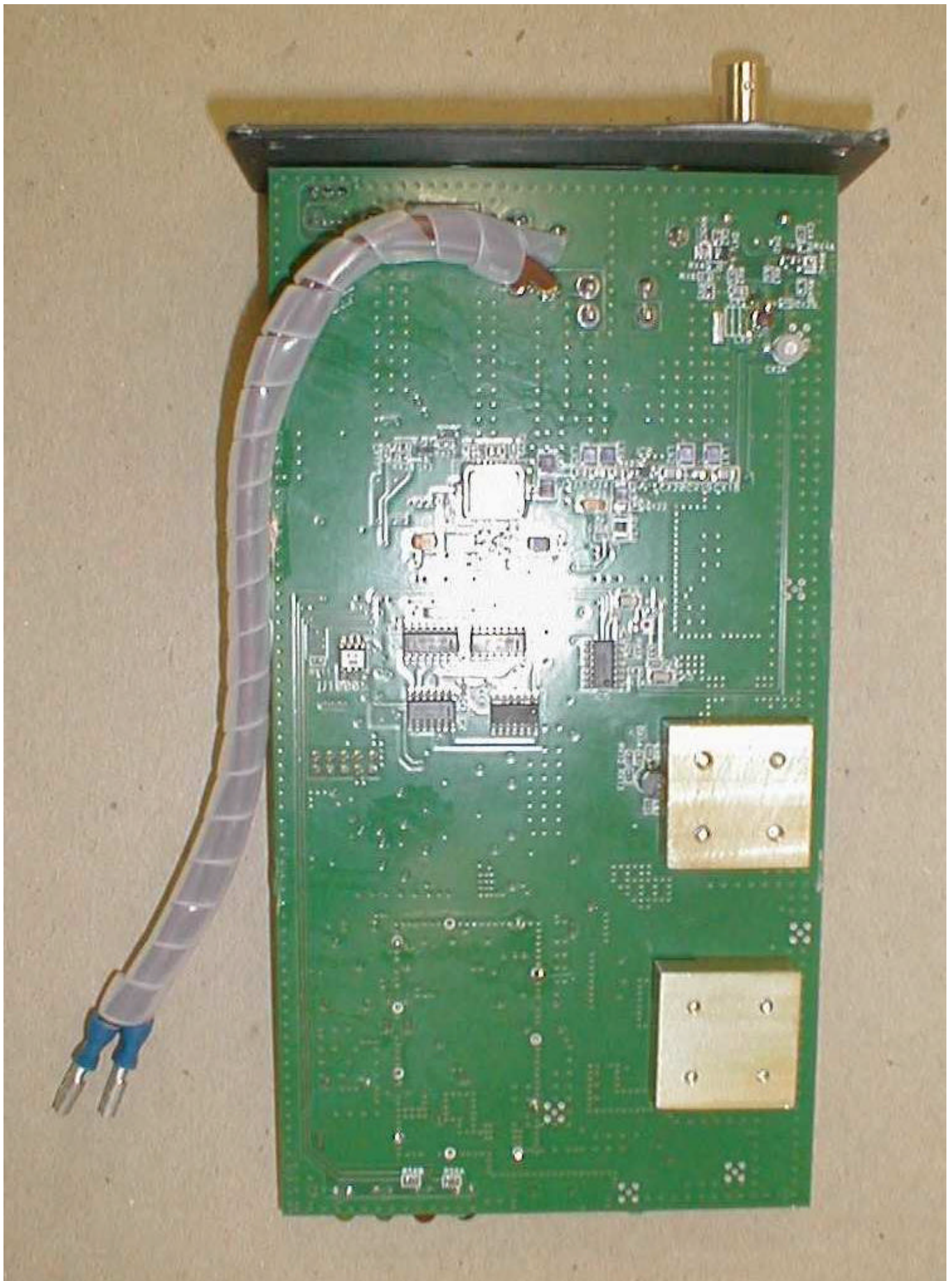
PCB Bottom
