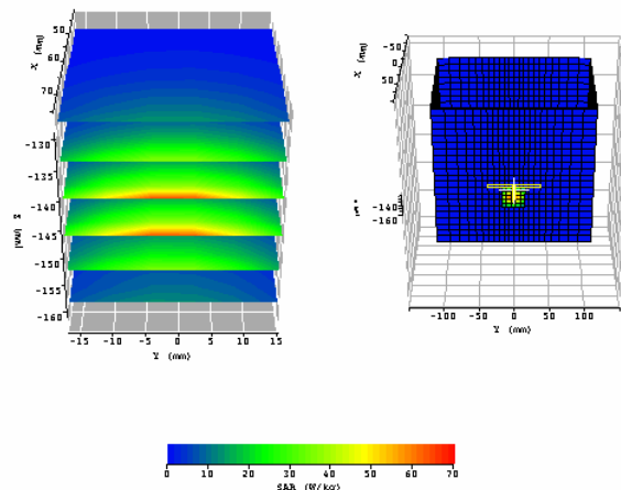
2450 MHz
