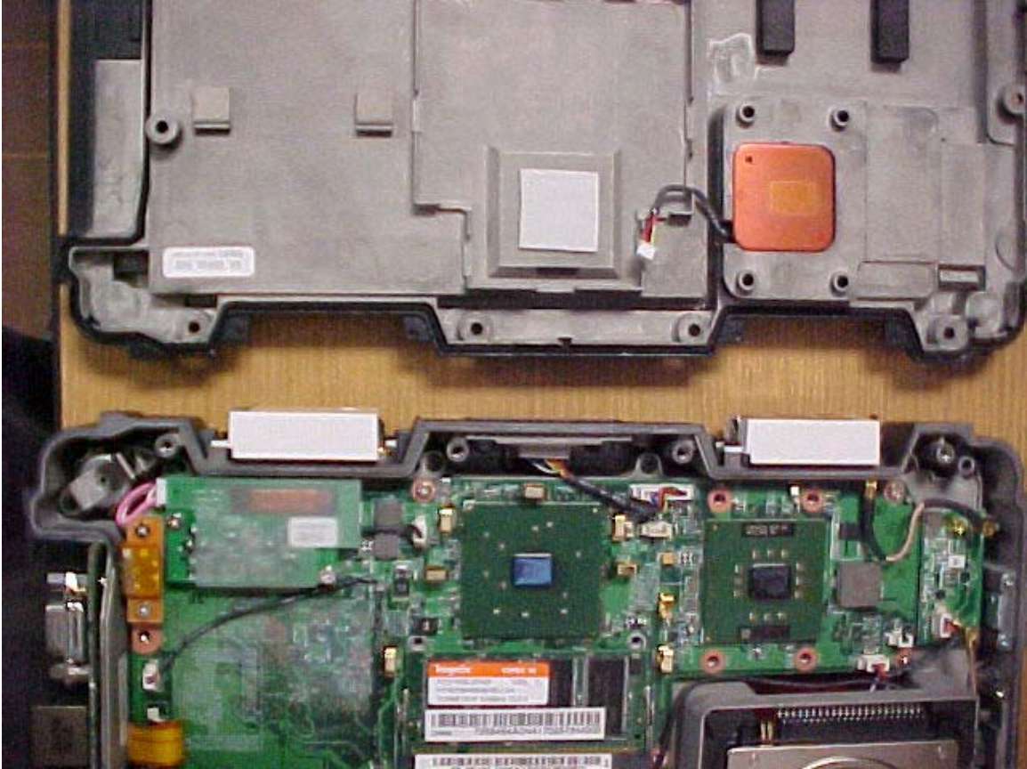
MVC-013F – PCB
