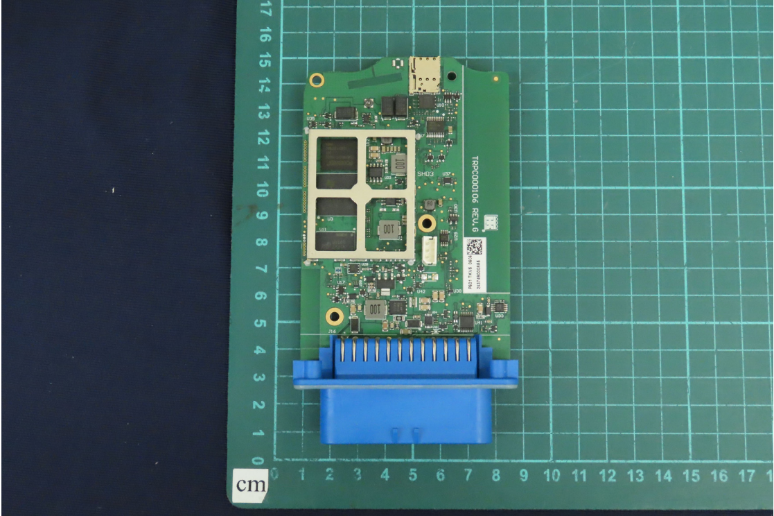
(8) EUT Photo
