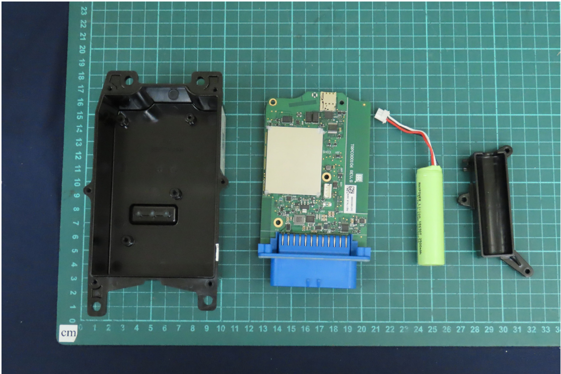
(3) EUT Photo
