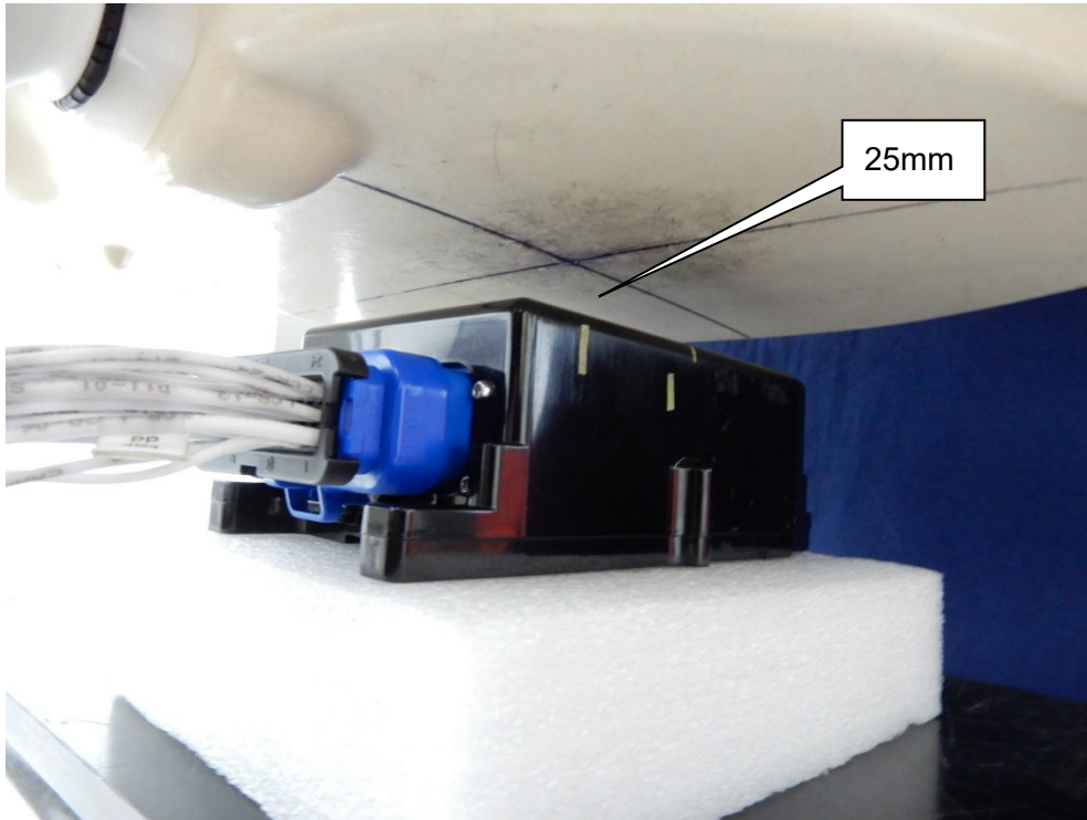
EUT Front_25mm
