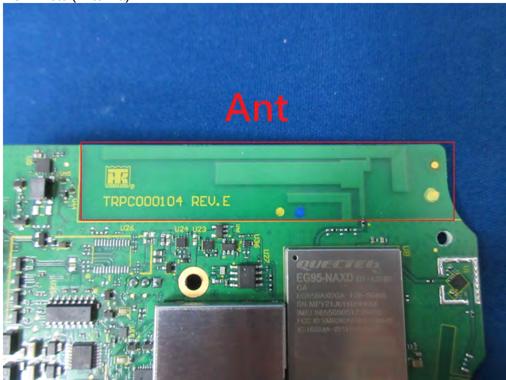
(6) EUT Photo (Antenna)
