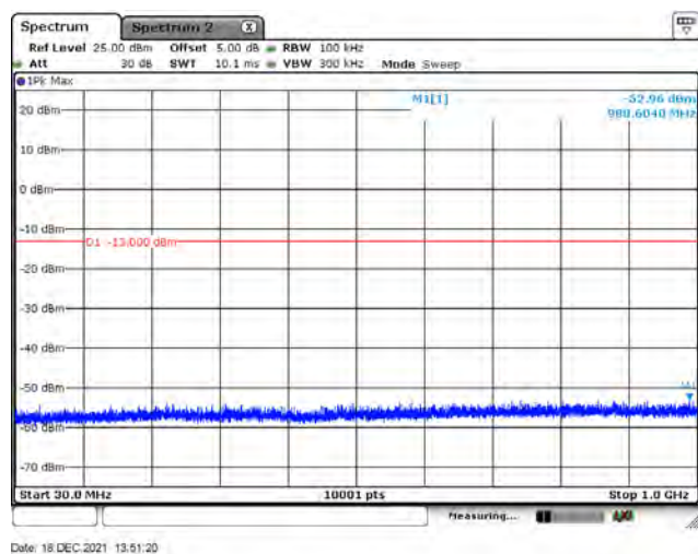
WCDMA Band 4 / RMC / 1732.6 MHz (Below 1GHz)
