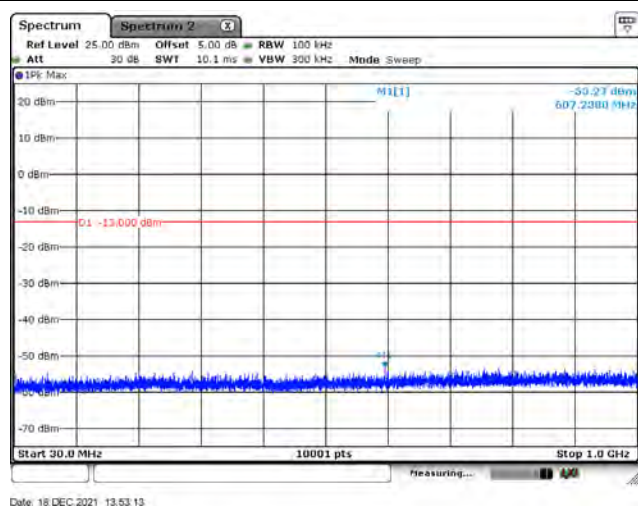
WCDMA Band 4 / RMC / 1752.6 MHz (Below 1GHz)
