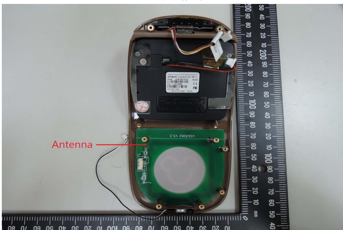
RFID Antenna
