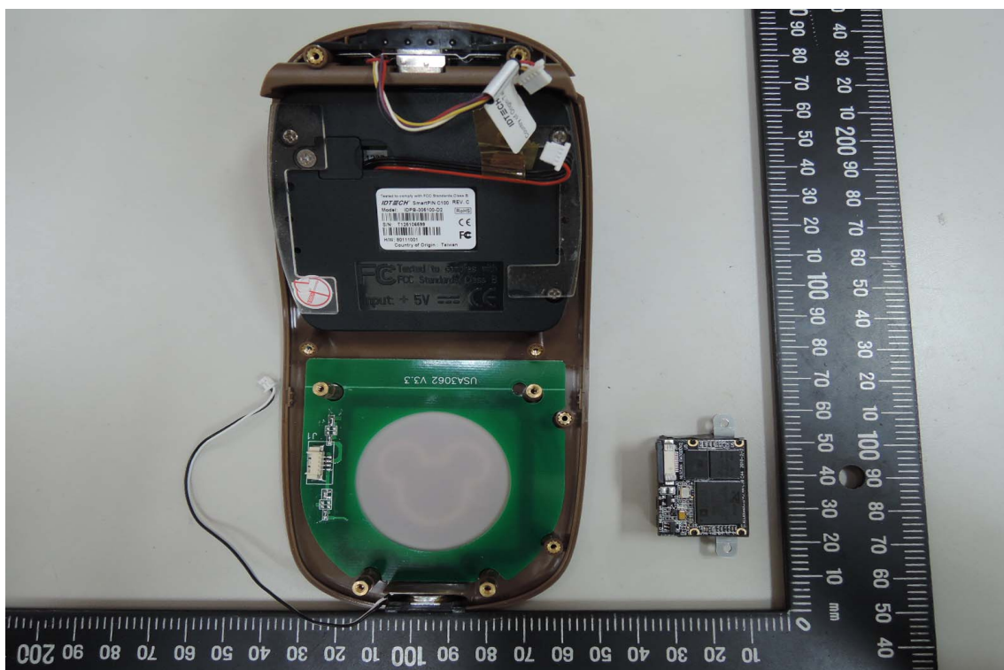
RFID Antenna
