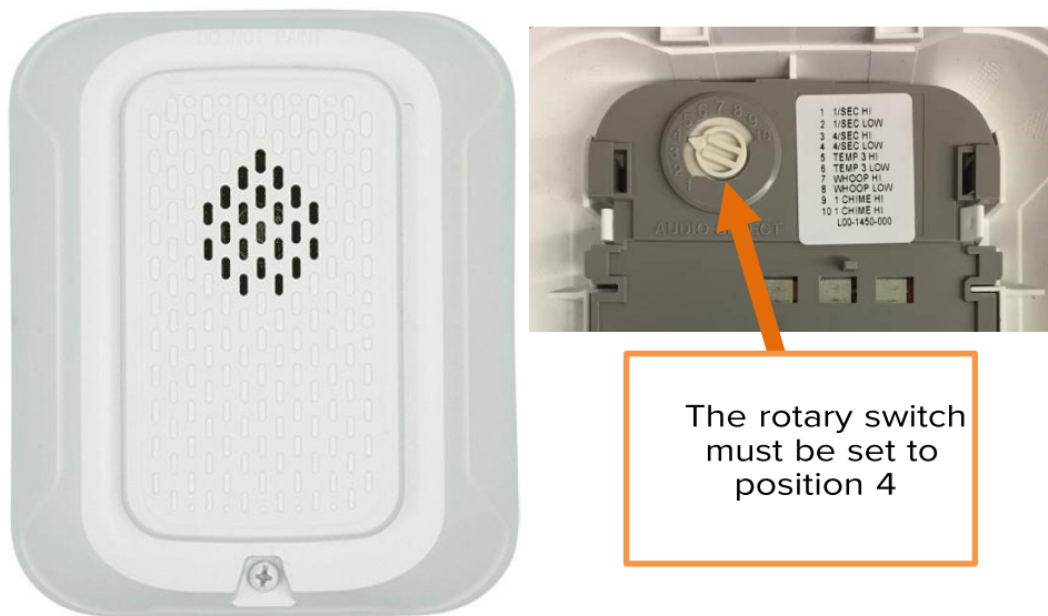
Figure 15. 56108 Siren
