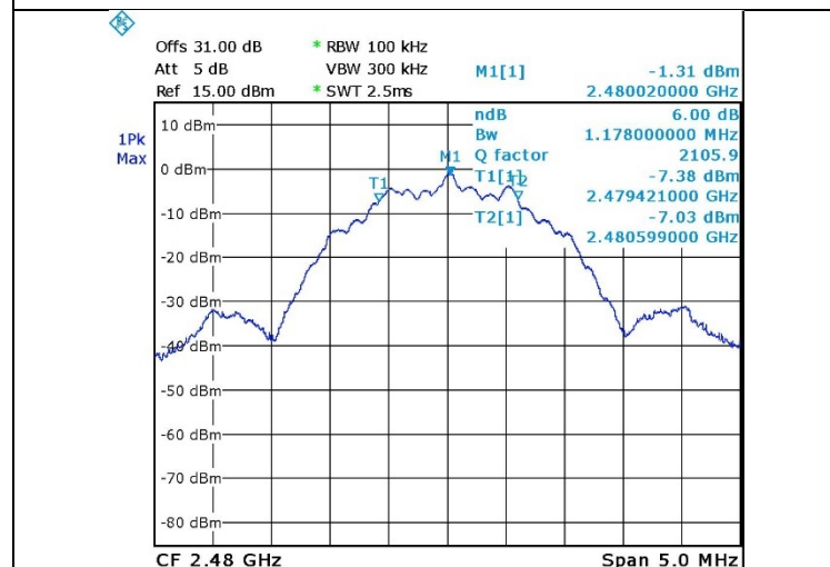
Figure 16. 2480.0 MHz, BLE
