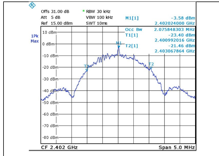
Figure 33. 2402.0 MHz, BLE
