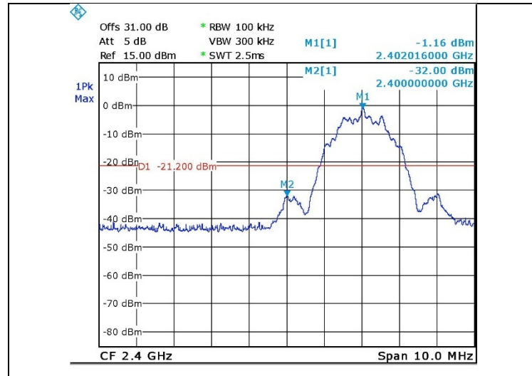
Figure 24. 2402.0 MHz, BLE
