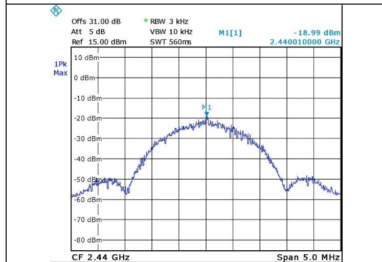
Figure 29. 2440.0 MHz, BLE
