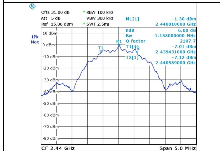
Figure 15. 2440.0 MHz, BLE
