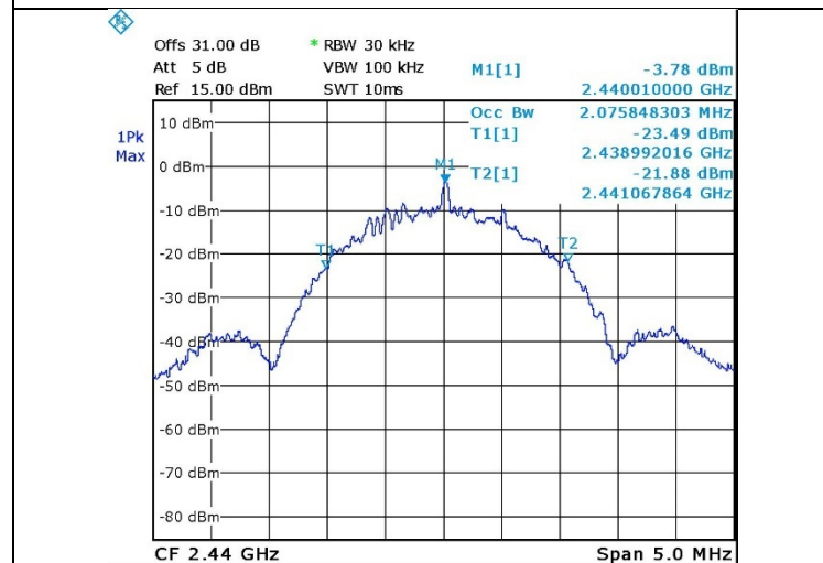
Figure 34. 2440.0 MHz, BLE
