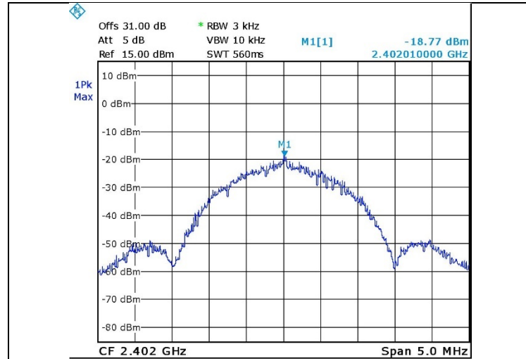
Figure 28. 2402.0 MHz, BLE
