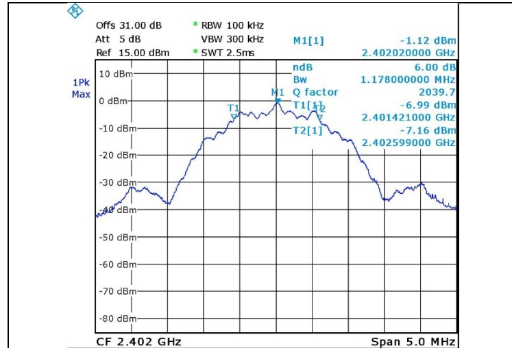
Figure 14. 2402.0 MHz, BLE
