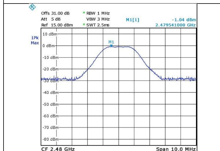
Figure 21. 2480.0 MHz, BLE
