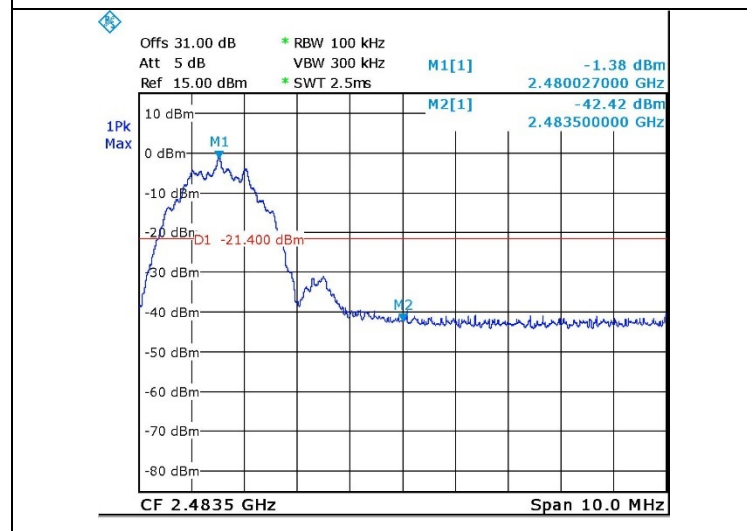
Figure 25. 2480.0 MHz, BLE
