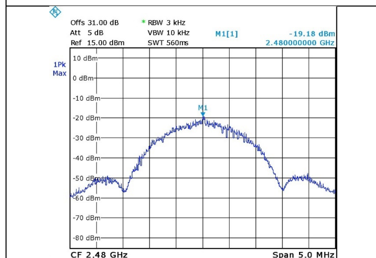
Figure 30. 2480.0 MHz, BLE
