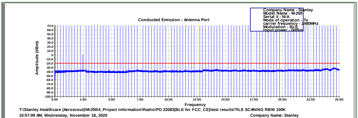
Figure 39 2480.0 MHz, BLE
