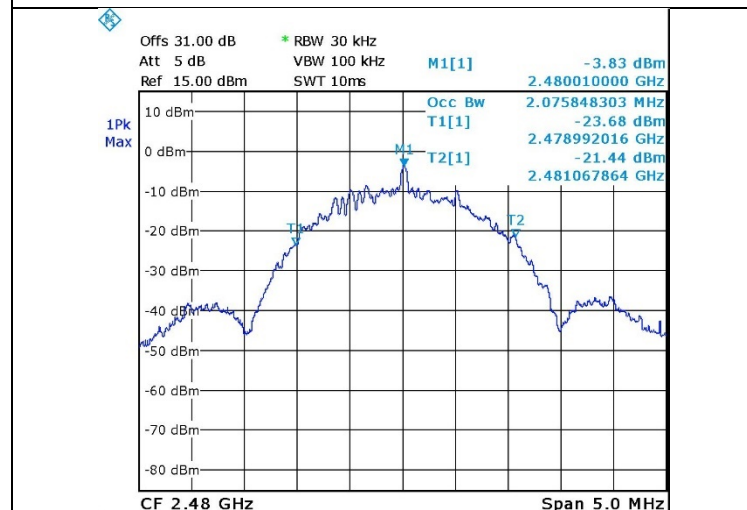
Figure 35. 2480.0 MHz, BLE
