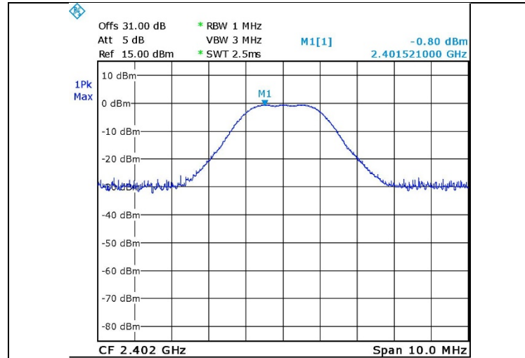
Figure 19. 2402.0 MHz, BLE
