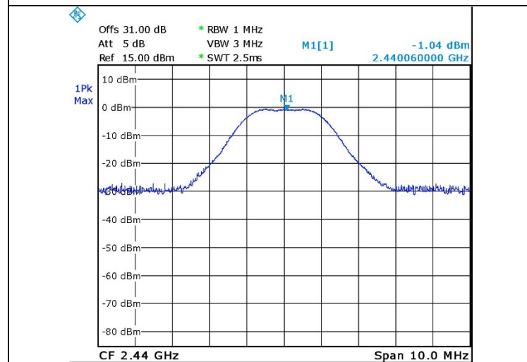
Figure 20. 2440.0 MHz, BLE
