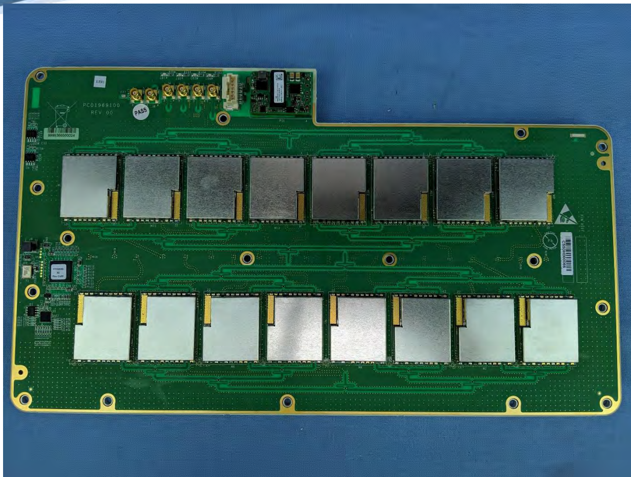
Upper Array Back
