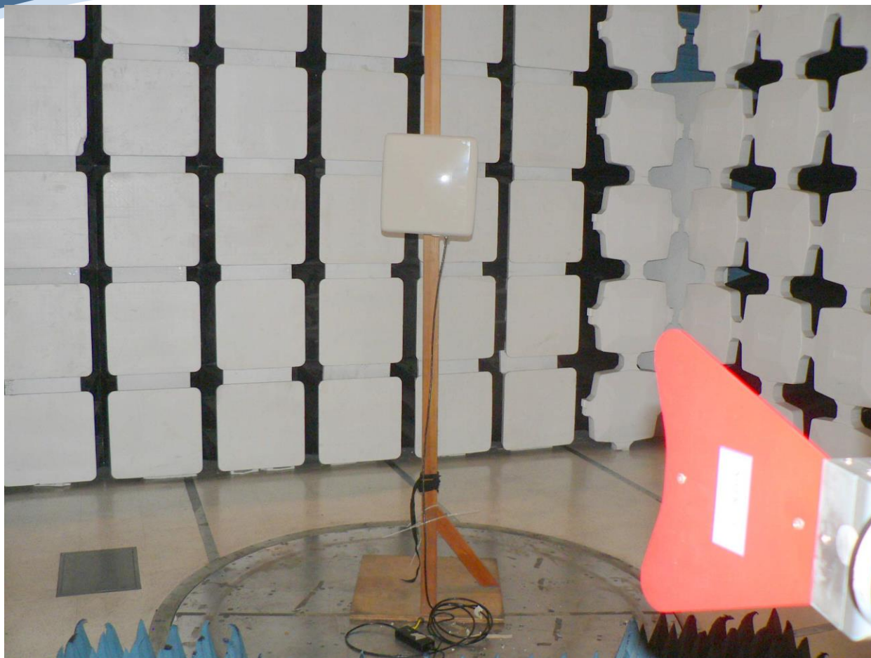
RDWN64 TX Spurious 1-18GHz
