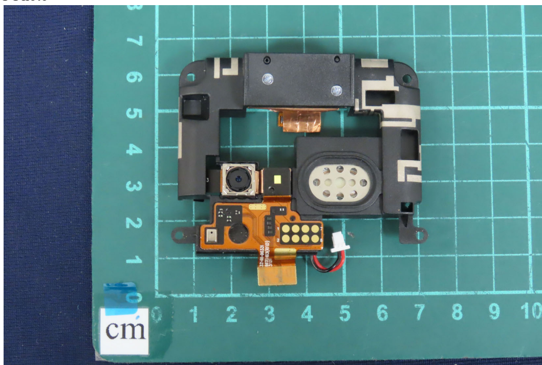
(21) EUT Photo
