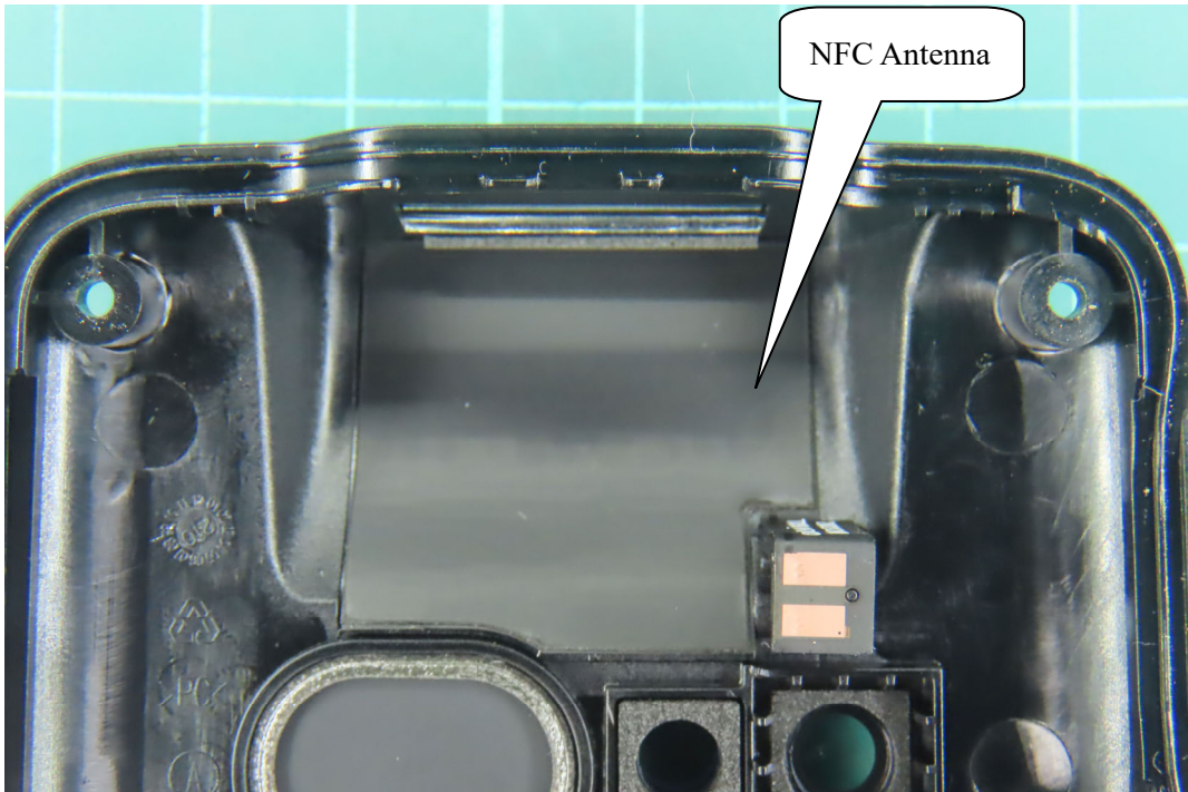
(14) EUT Photo
