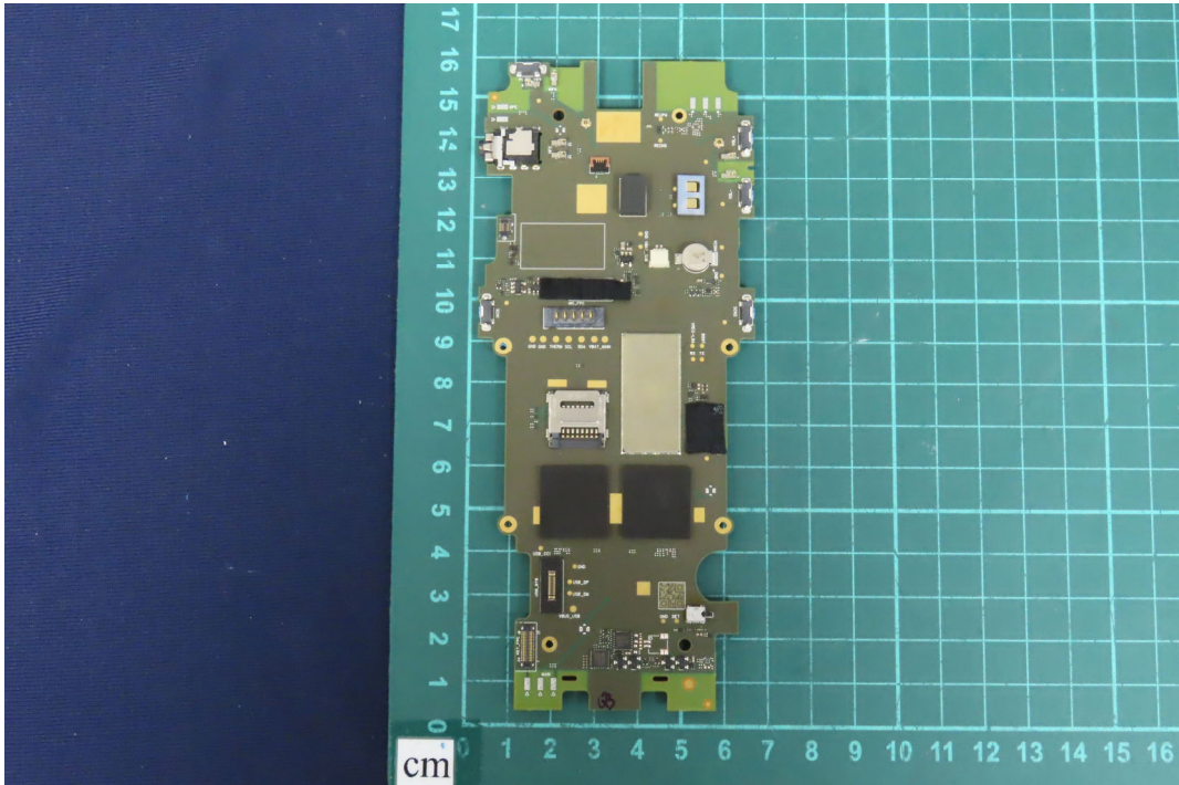
(31) EUT Photo
