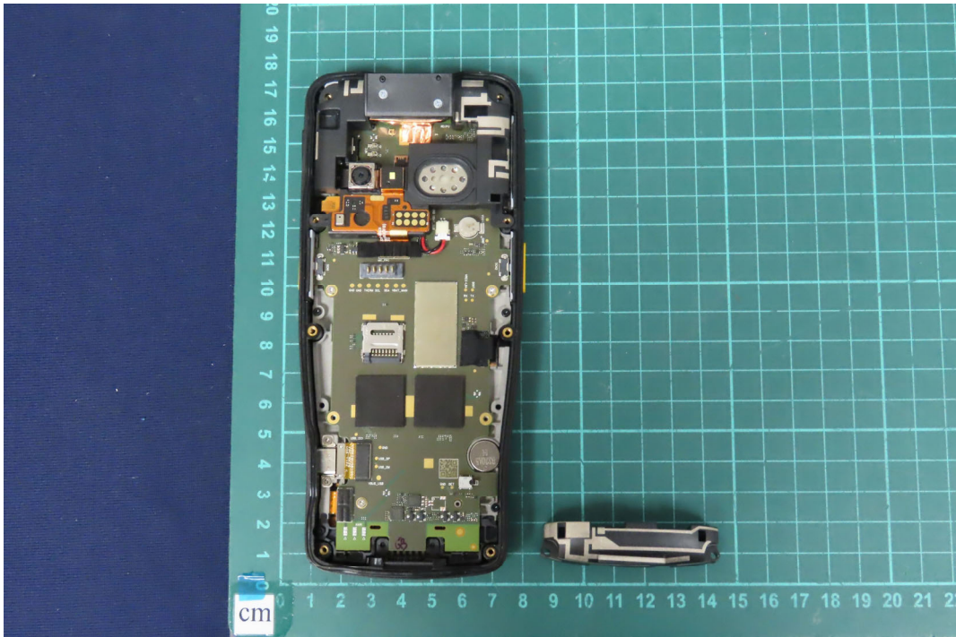
(16) EUT Photo
