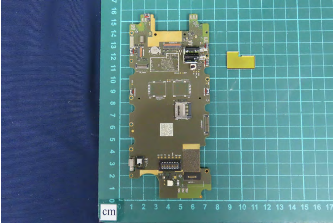
(20) EUT Photo
