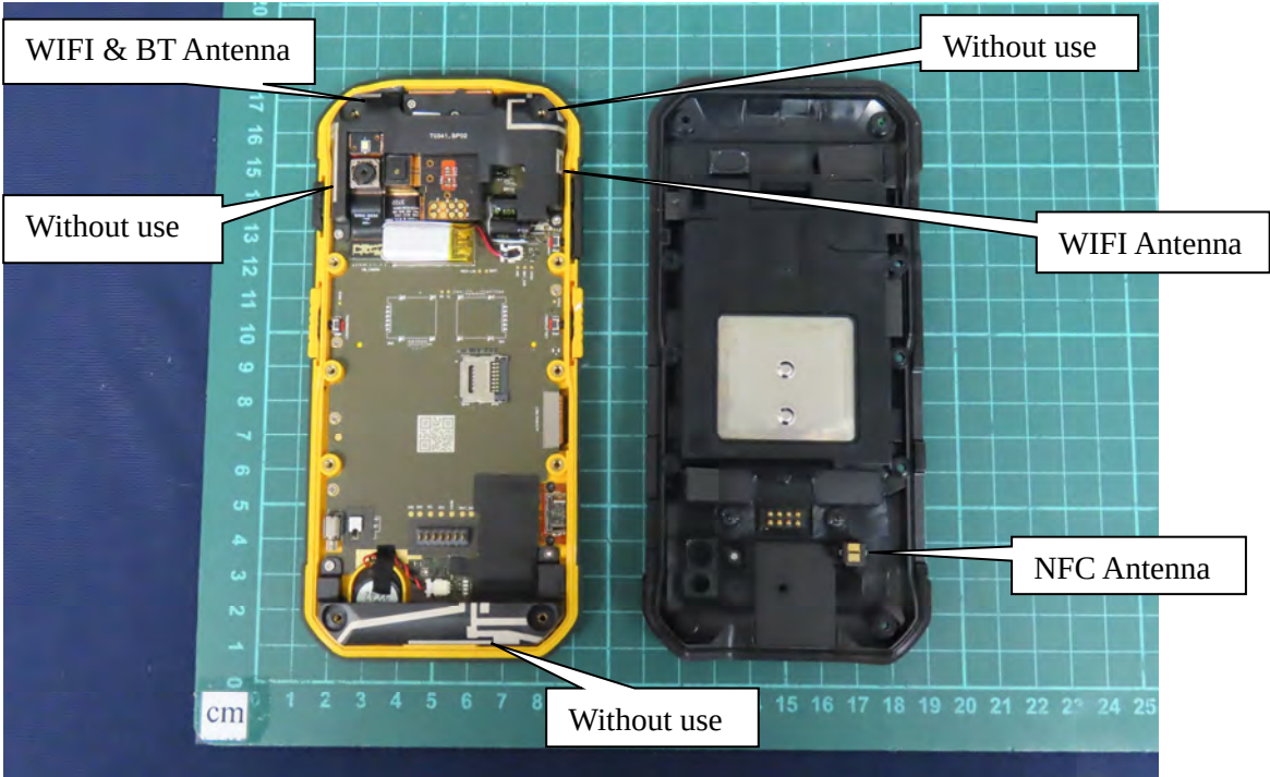
(5) EUT Photo
