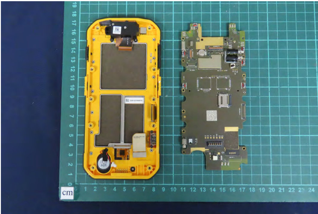
(18) EUT Photo
