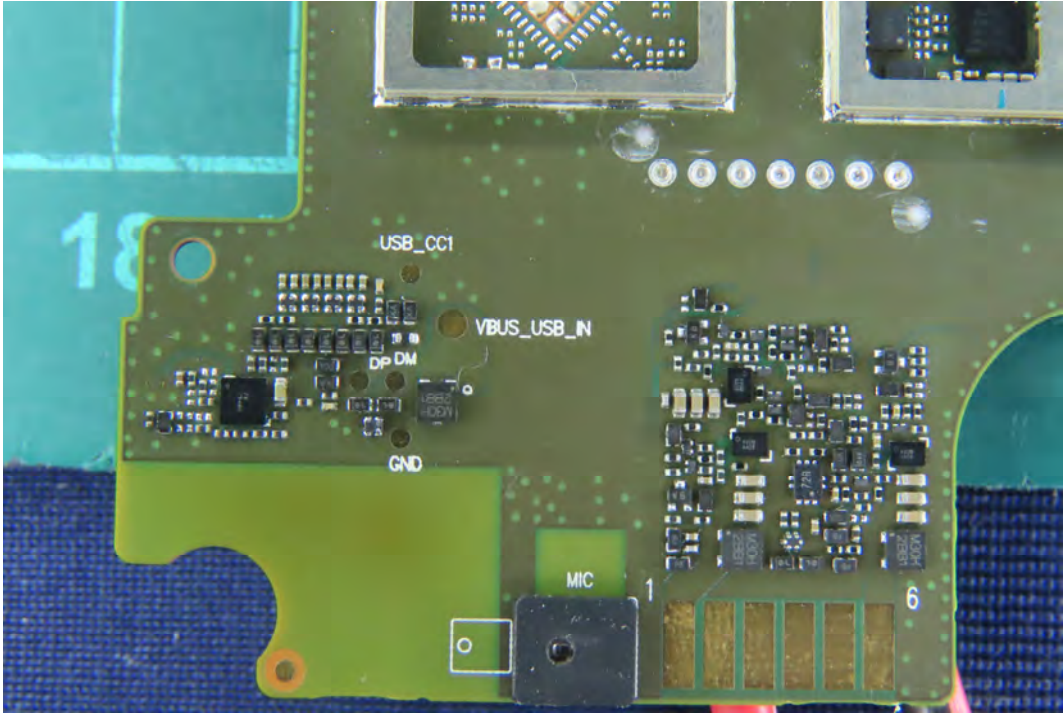
(30) EUT Photo
