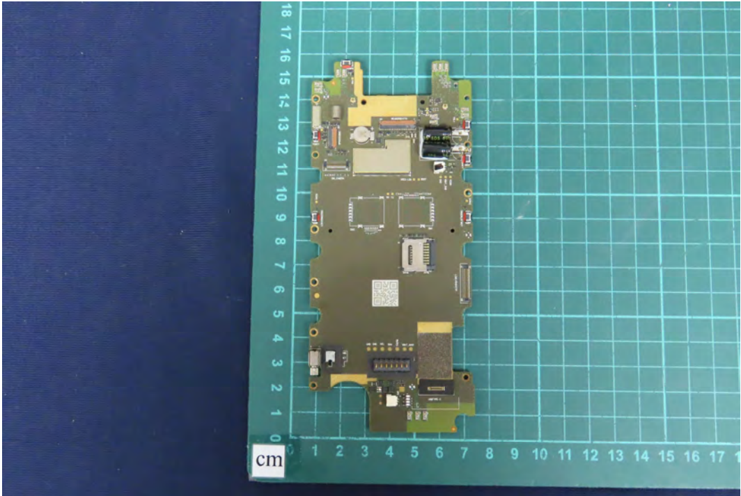
(19) EUT Photo
