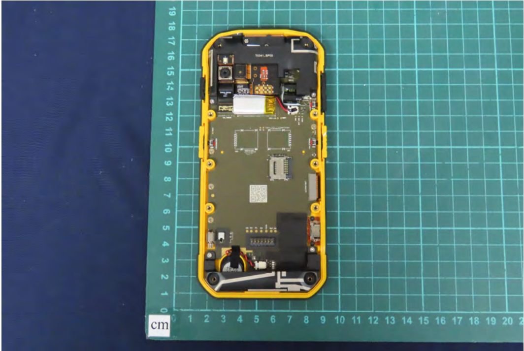
(6) EUT Photo
