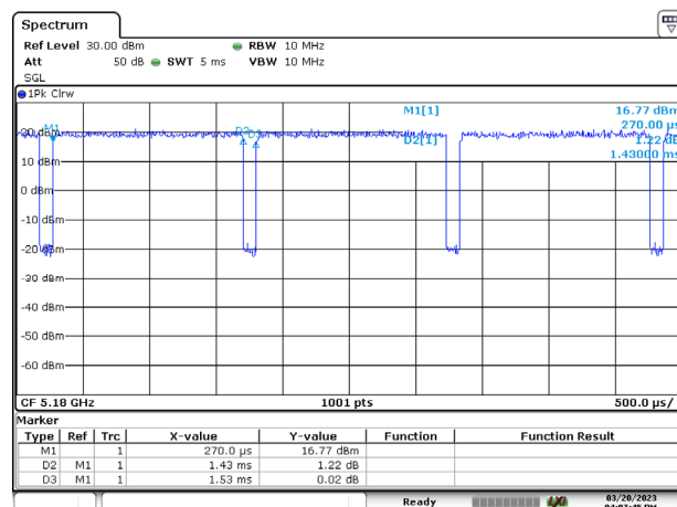
802.11a
