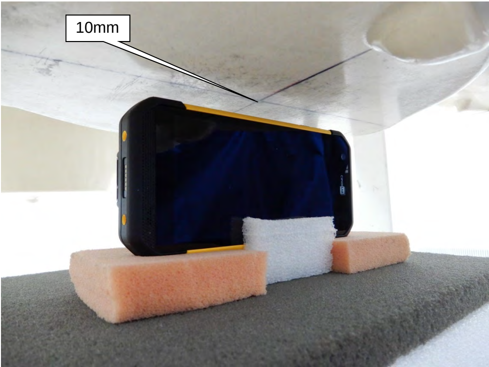
EUT Left-side_10mm
