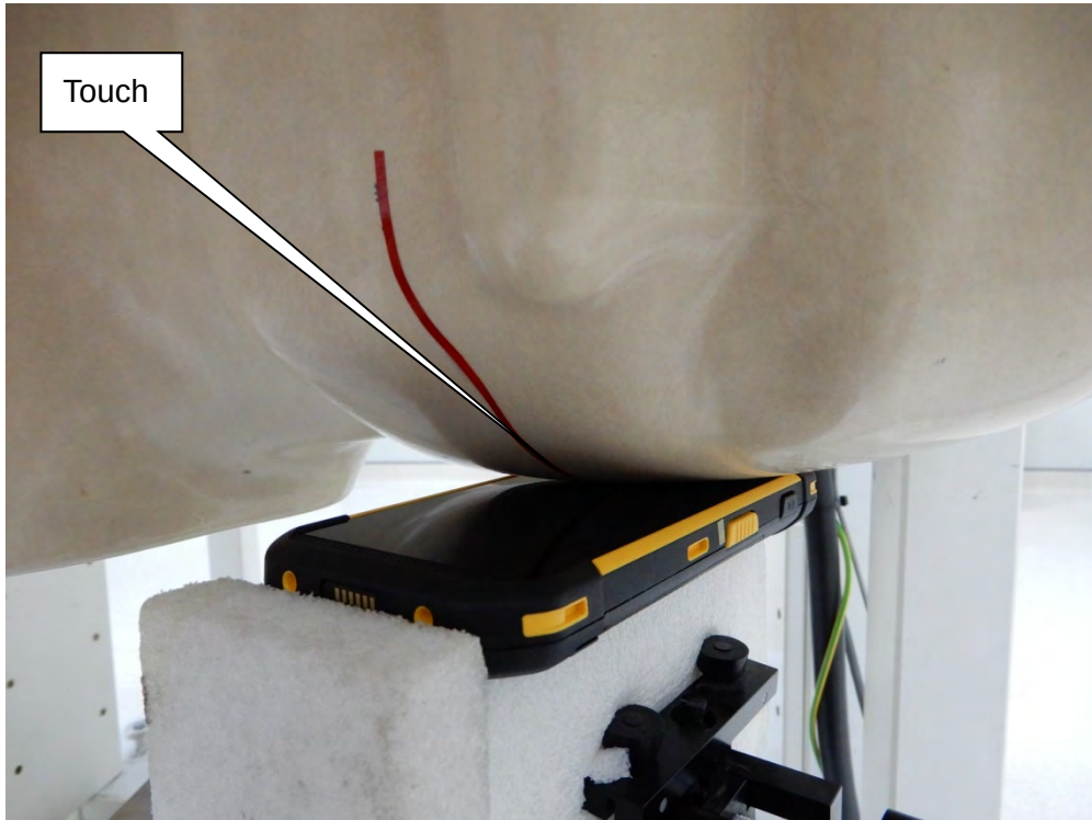
EUT Left-Cheek
