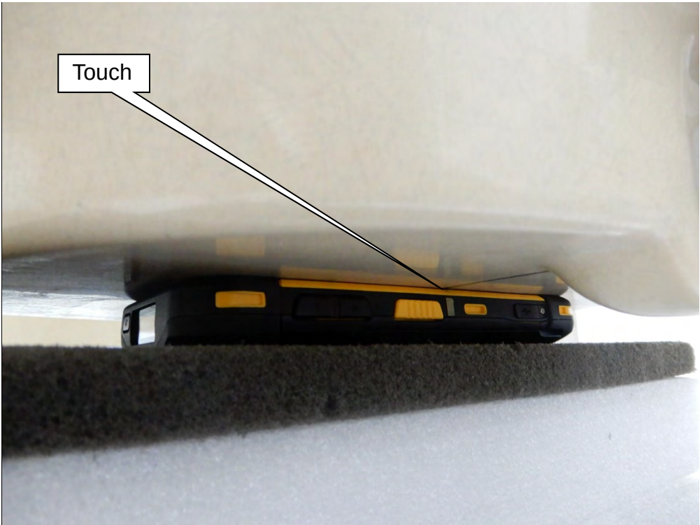
EUT Front_0mm
