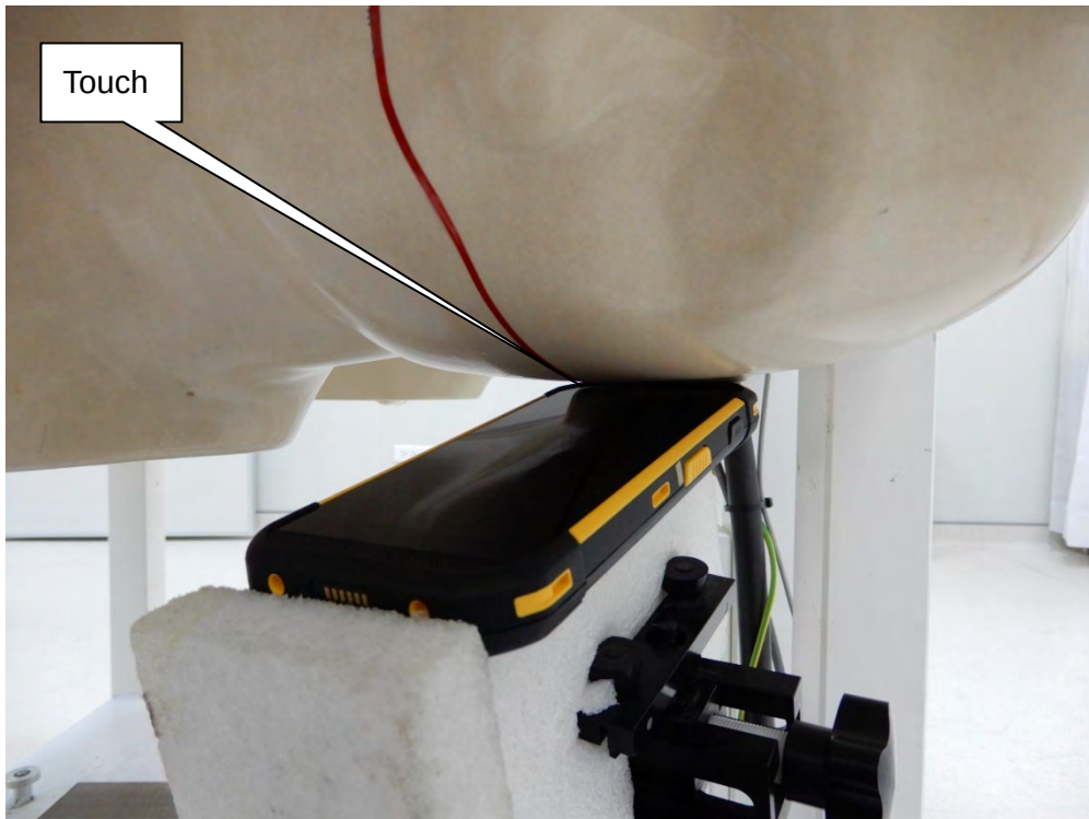
EUT Left-Tilt
