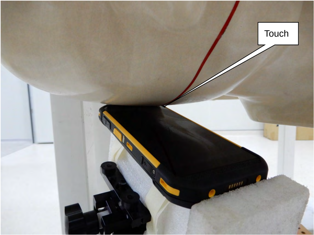
EUT Right-Tilt
