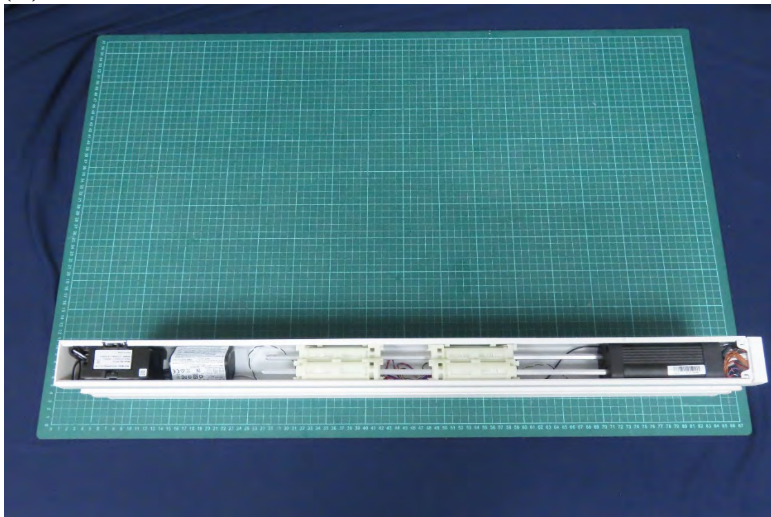
(14) EUT Photo_DMCS1-B
