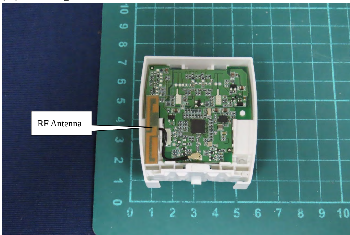
(18) EUT Photo_DMCS1-B
