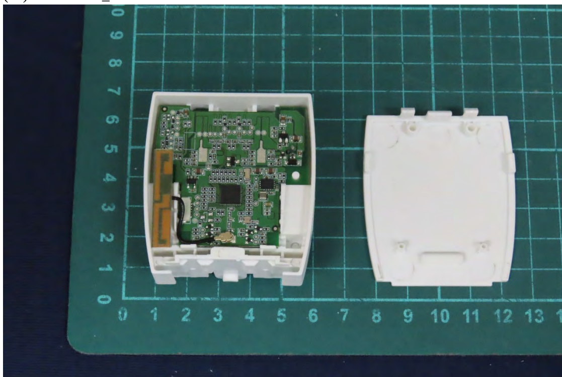
(17) EUT Photo_DMCS1-B
