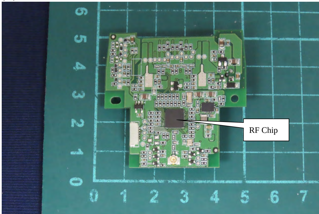
(22) EUT Photo_DMCS1-B
