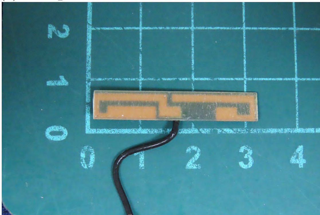
(21) EUT Photo_DMCS1-B
