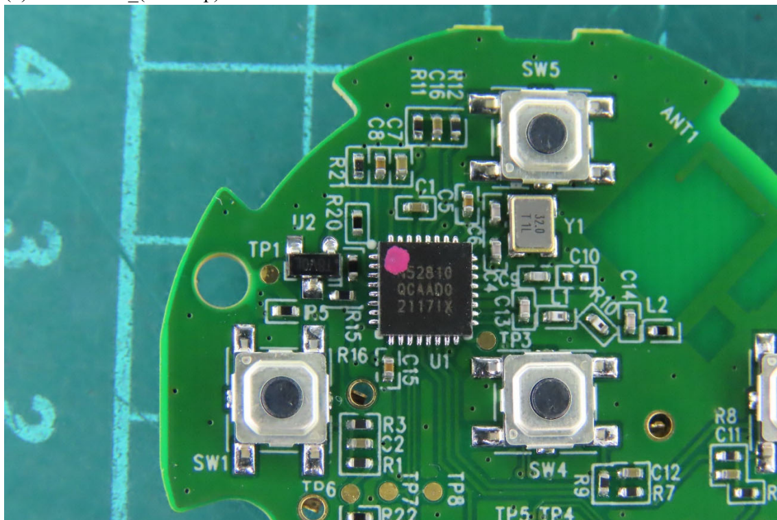
(7) EUT Photo_(RF Chip)
