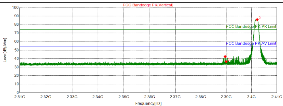
BLE_2402_Ant1/ Vertical
