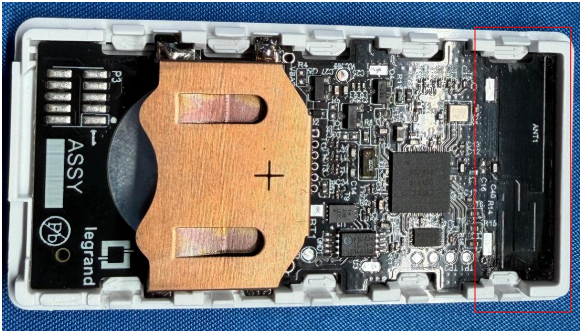
Antenna
