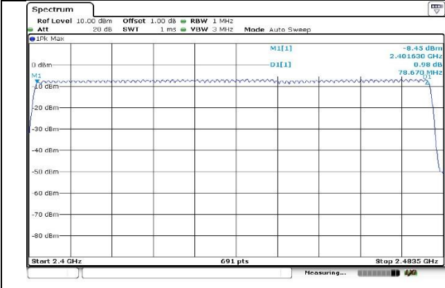
8DPSK
