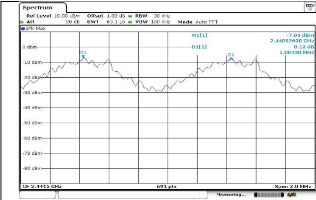
GFSK
