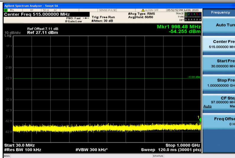
Band25-20MHz-QPSK-26140-1RB#0-30~1000MHz
