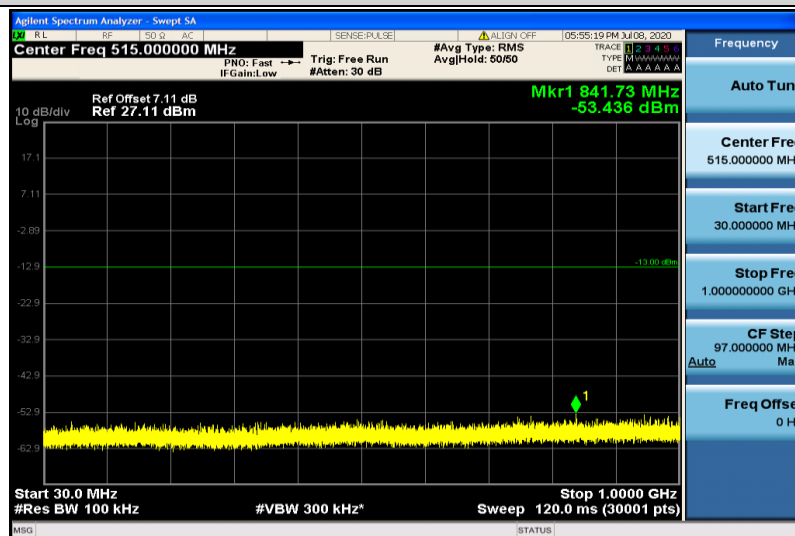
Band25-20MHz-QPSK-26590-1RB#0-30~1000MHz
