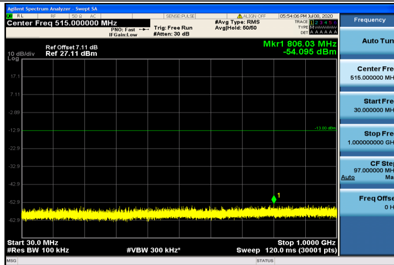
Band25-20MHz-QPSK-26365-1RB#0-30~1000MHz
