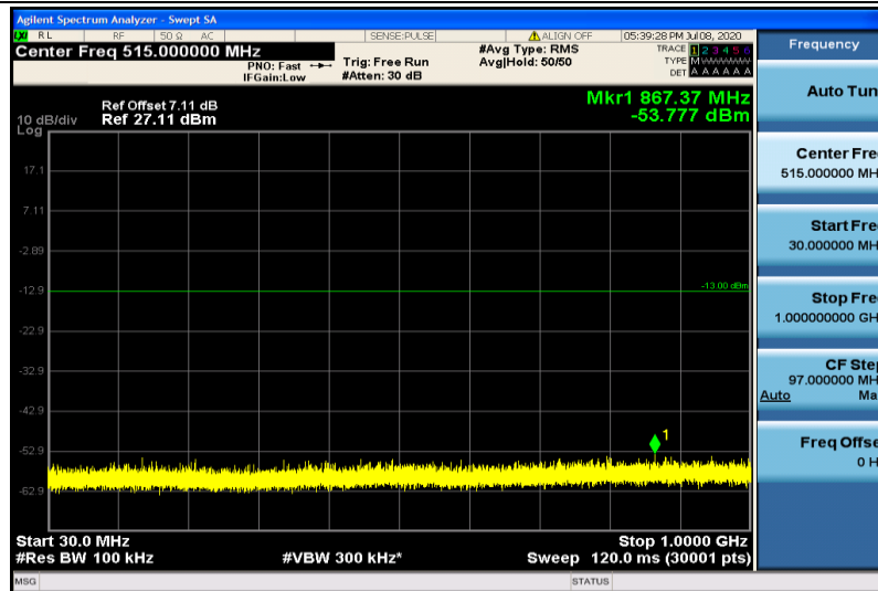
Band25-10MHz-QPSK-26365-1RB#0-30~1000MHz
