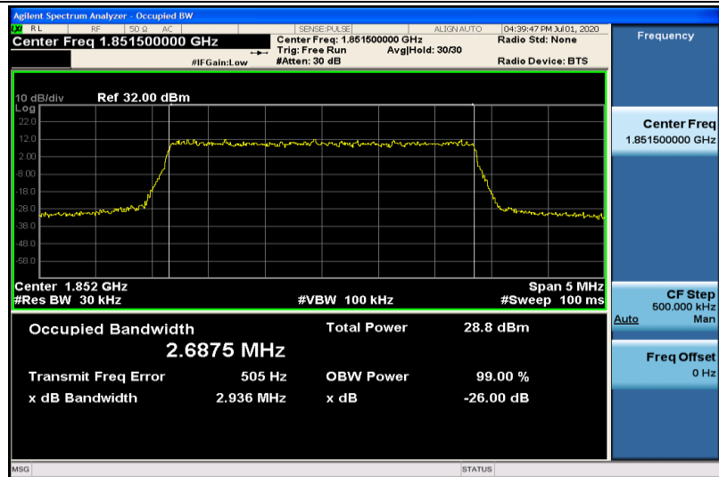
Band2-3MHz-QPSK-18615-15RB#0-2.6875
