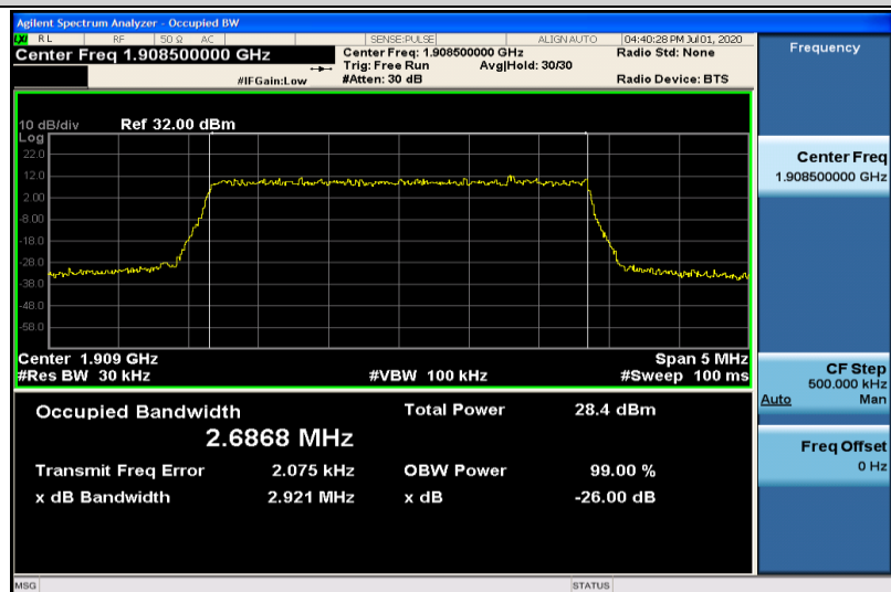
Band2-3MHz-QPSK-19185-15RB#0-2.6868
