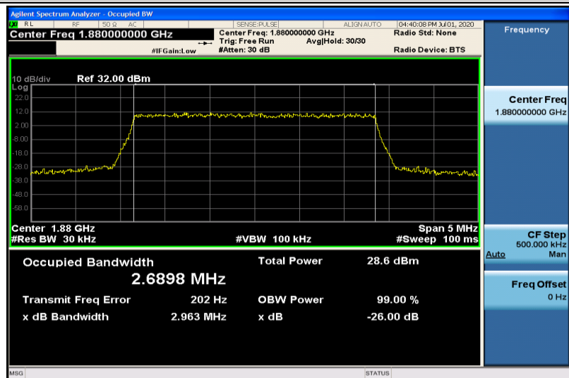
Band2-3MHz-QPSK-18900-15RB#0-2.6898
