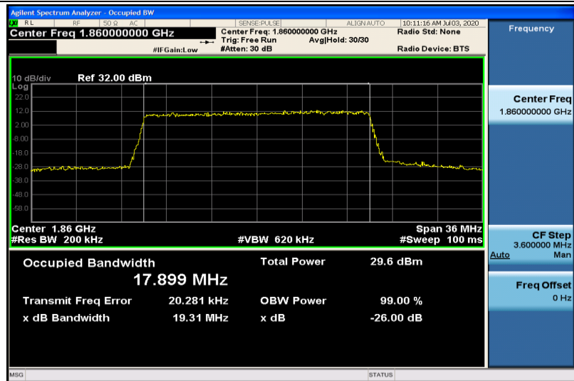
Band2-20MHz-QPSK-18700-100RB#0-17.899
