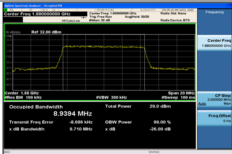
Band2-10MHz-QPSK-18900-50RB#0-8.9394
