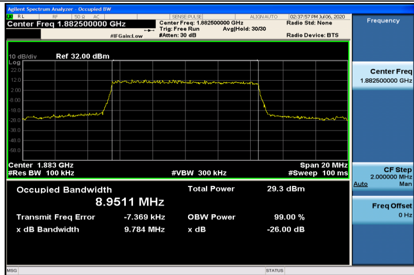
Band25-10MHz-QPSK-26365-50RB#0-8.9511
