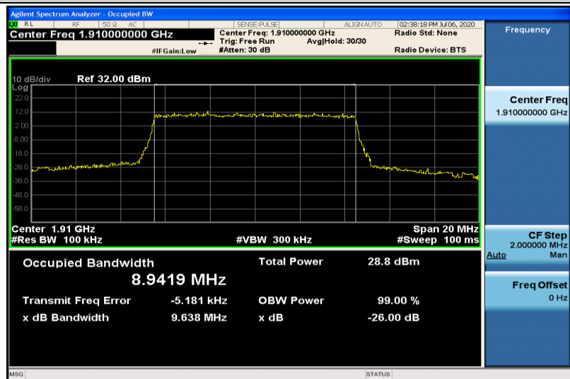
Band25-10MHz-QPSK-26640-50RB#0-8.9419
