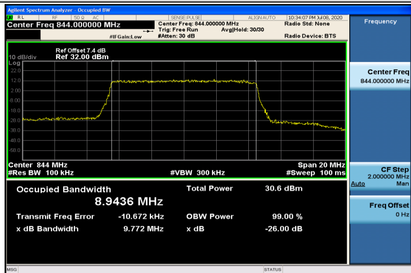
Band26-10MHz-QPSK-26990-50RB#0-8.9436
