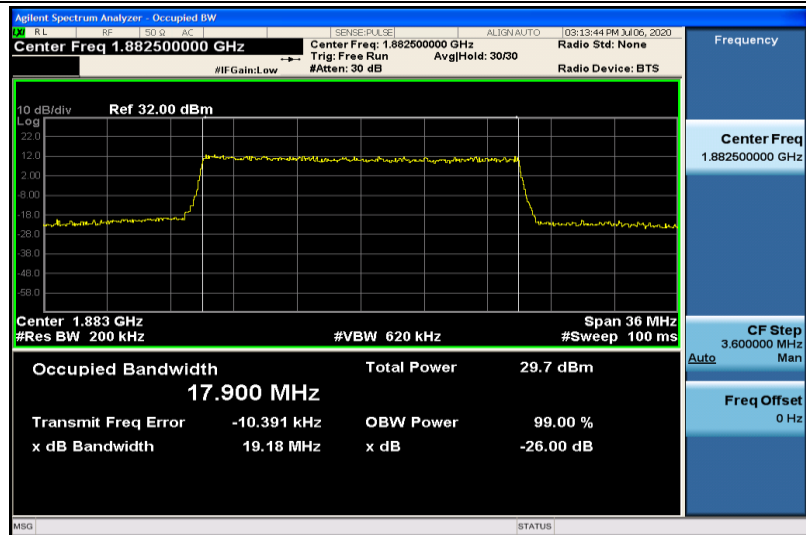
Band25-20MHz-QPSK-26365-100RB#0-17.900
