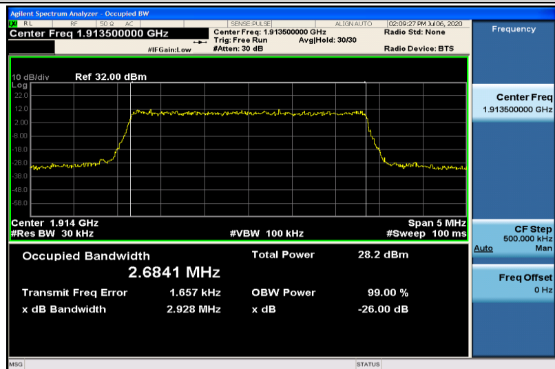
Band25-3MHz-QPSK-26675-15RB#0-2.6841
