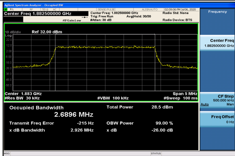
Band25-3MHz-QPSK-26365-15RB#0-2.6896
