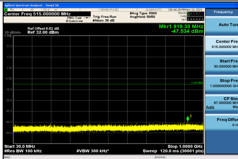
Band2-20MHz-QPSK-18900-1RB#0-30~1000MHz
