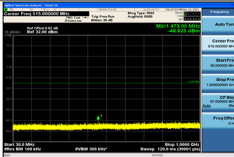
Band2-20MHz-16QAM-18900-1RB#0-30~1000MHz
