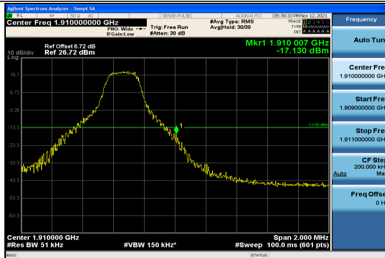
Band2-5MHz-QPSK-19175-1RB#24
