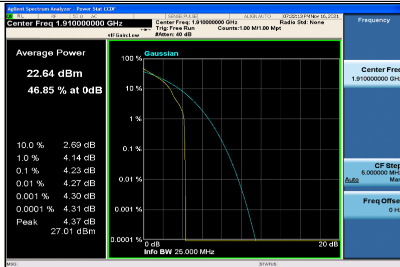
Band25-10MHz-QPSK-26640-1RB#0
